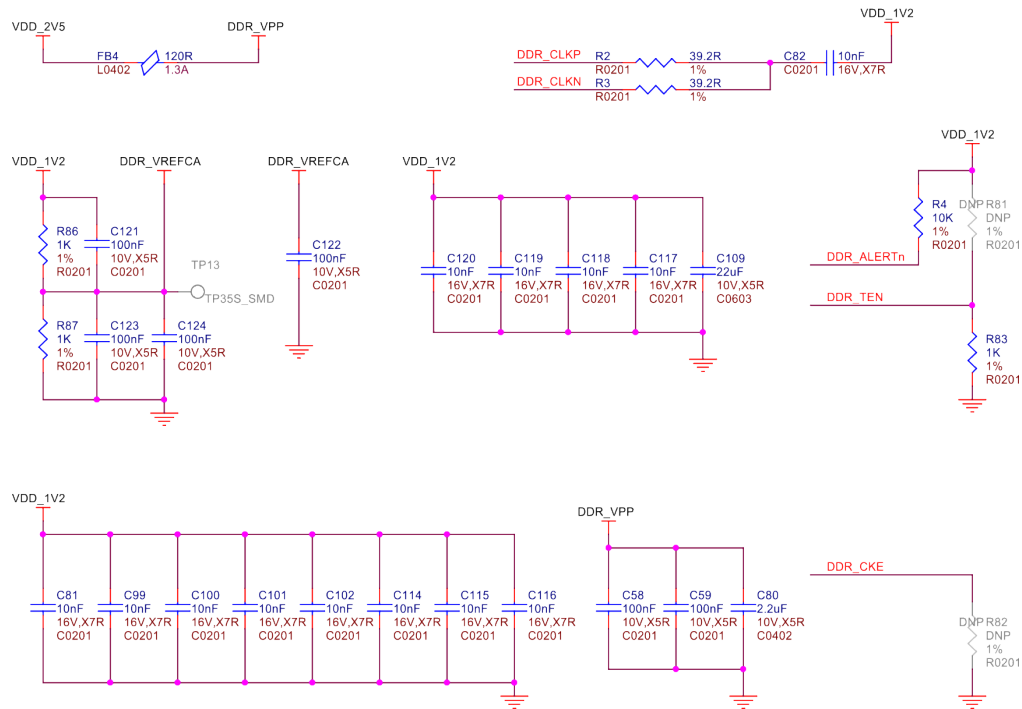
Fig. 3.40: DDR power
